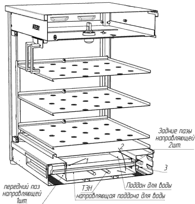
Рис.4 (в разрезе)
